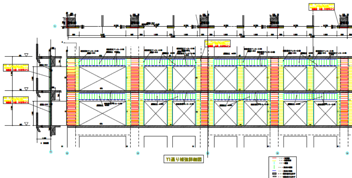
図 2.2 補強鉄筋割付図 6F. 7F ベランダ側
